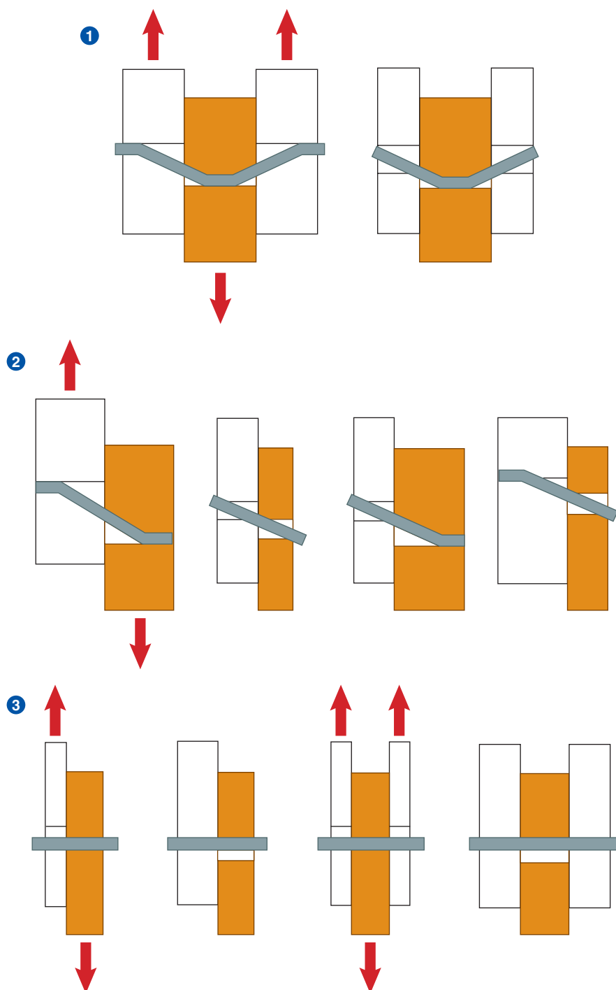
Figure 20 - Mode de rupture des assemblages en cisaillement : 1. Double cisaillement par plastification de l'acier. 2. Simple cisaillement avec plastification de l'acier. 3. Rupture par enfoncement dans le bois.
