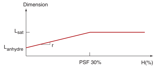
Figure 9 - Retrait du bois.
